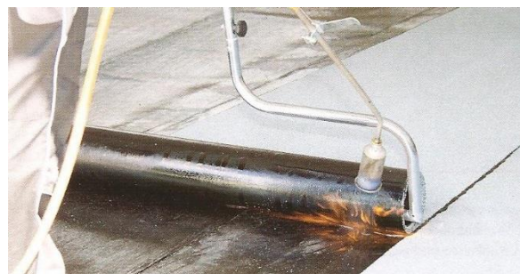
Variantní natavování rozbalovačem rolem
